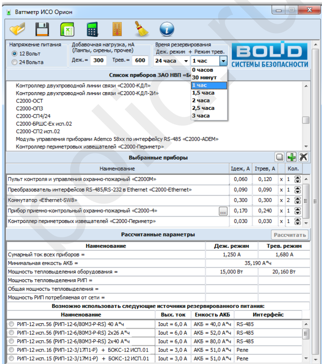
Интерфейс утилиты "Ваттметр ИСО Орион"
