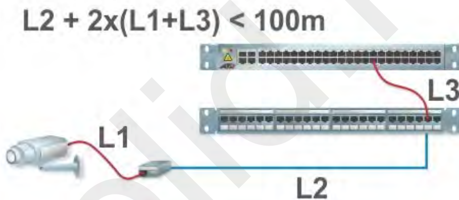
Составляющие 100 метров Ethernet
