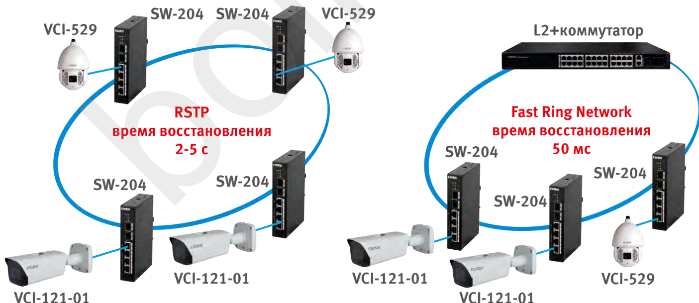
Кольцевая топология Ethernet
