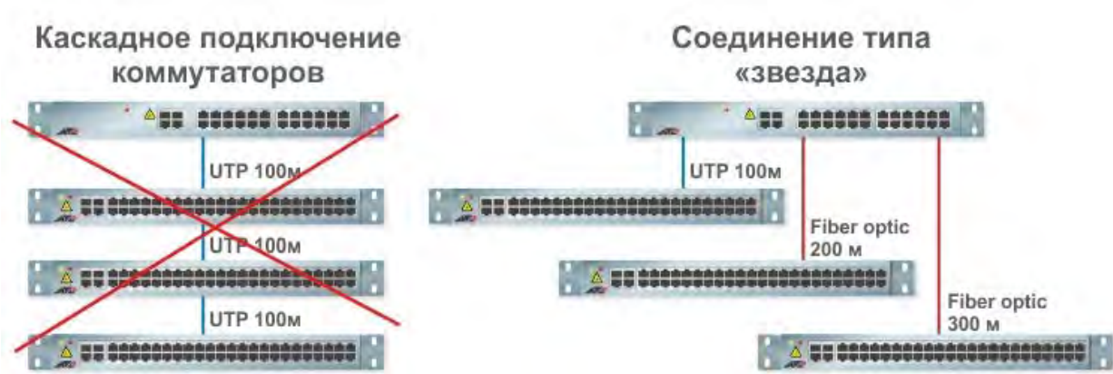
Древовидная топология Ethernet
