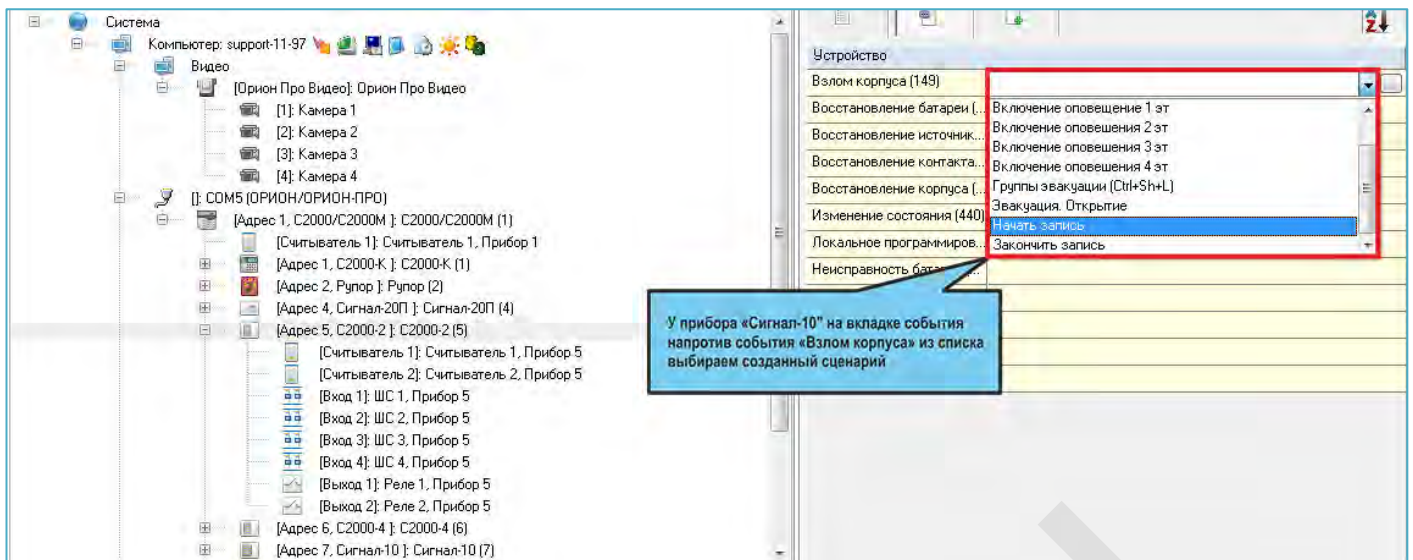
Привязка созданного сценария к конкретному прибору Болид
