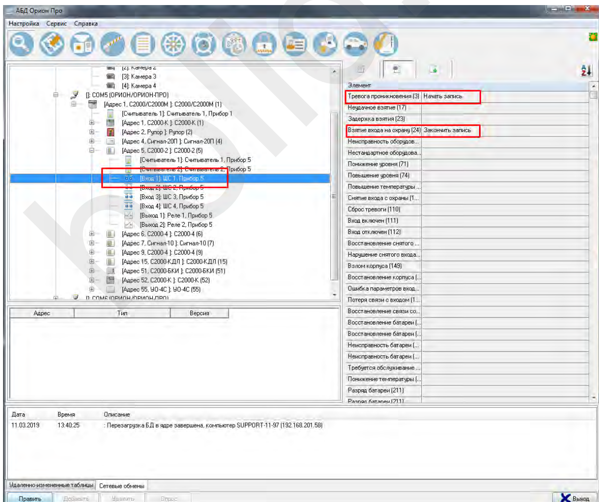
Настройка остановки записи после восстановления ШС
