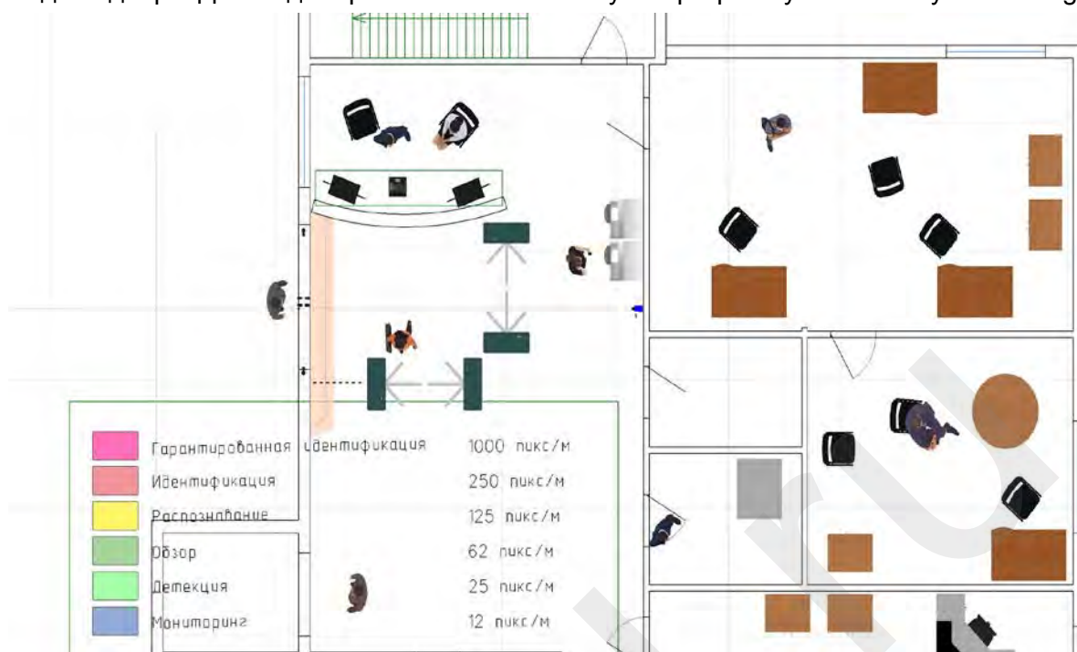
Пример выбора места установки видеокамеры и основных технических характеристик
