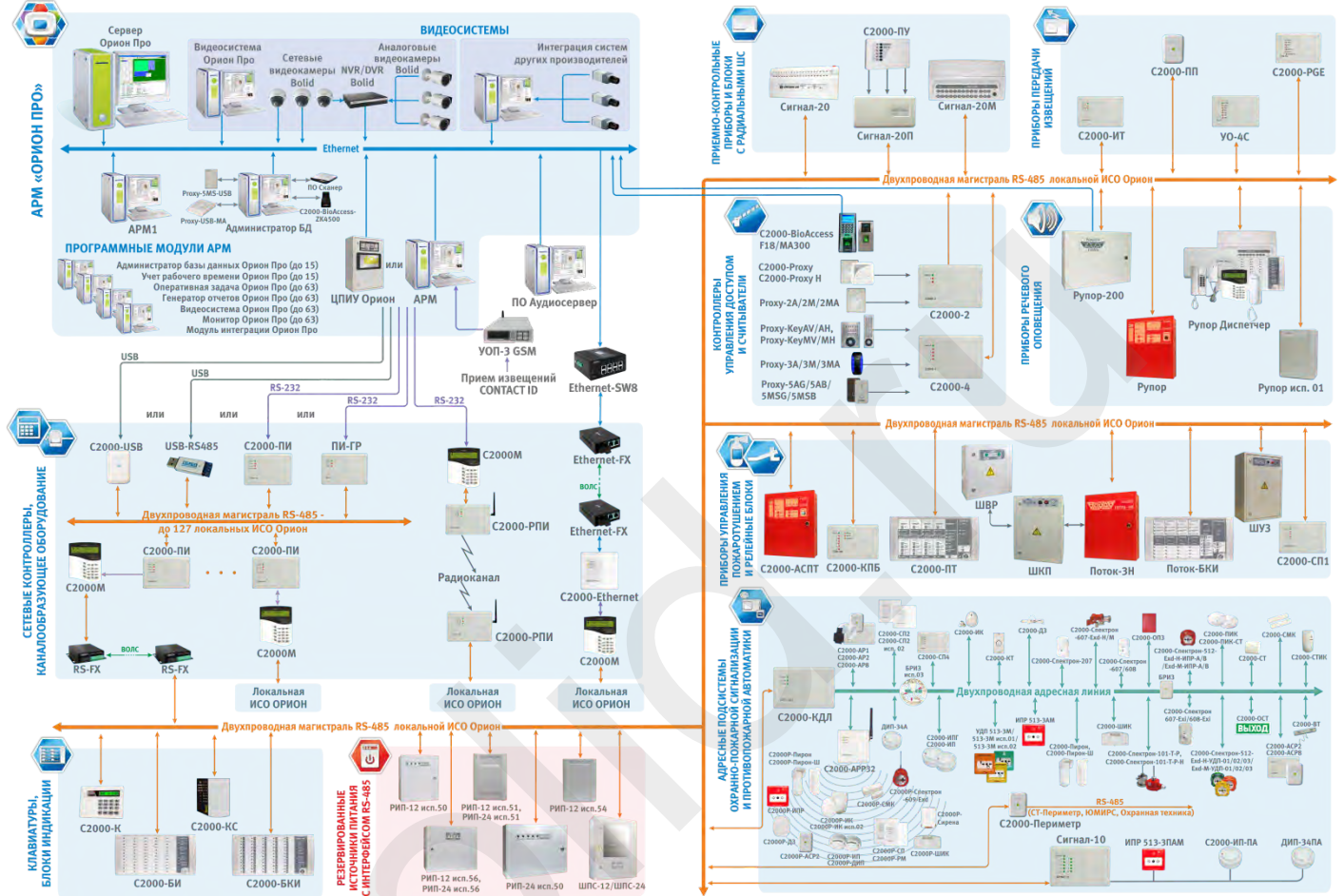
Структурная схема ИСО Орион - интегрированной системы безопасности
