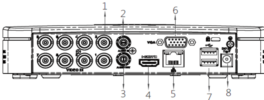
Рисунок 2 Внешний вид задней панели.
