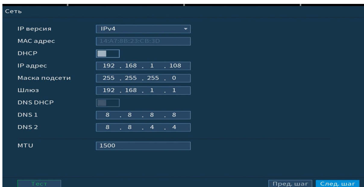
Рисунок 9 Интерфейс меню быстрой настройки «Сеть»
