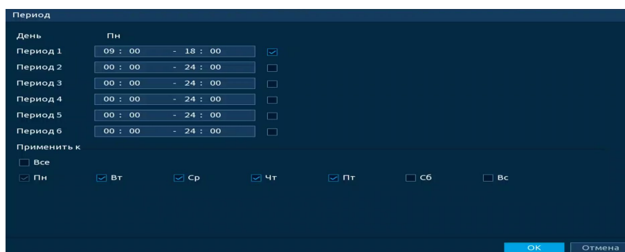
Рисунок 18.23 – Расписание
