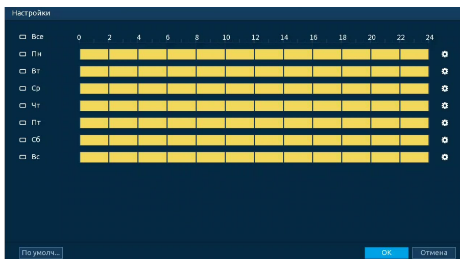
Рисунок 18.26 – Панель расписания
