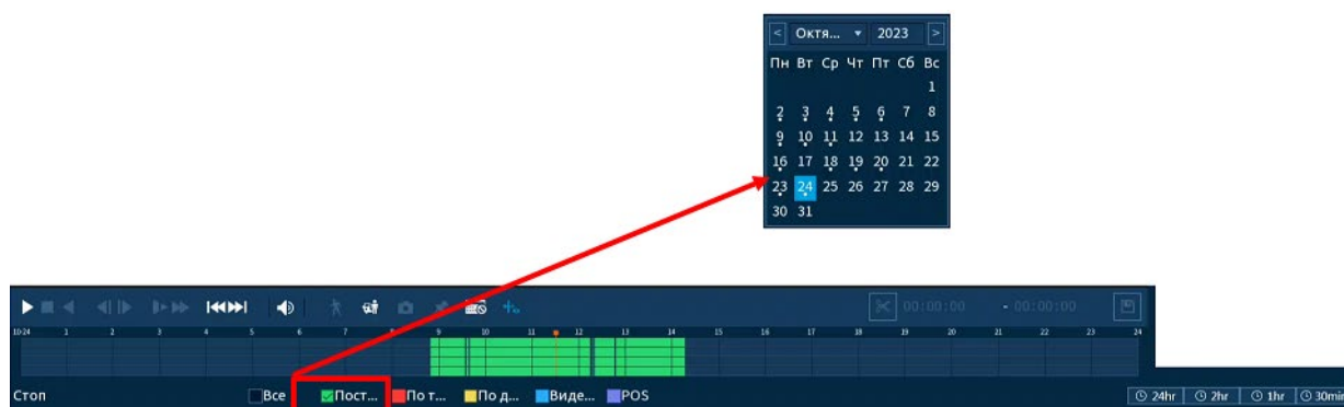
Рисунок 17.5 – Шкала времени
