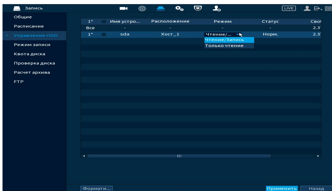
Рисунок 13.13 – Интерфейс настройки
