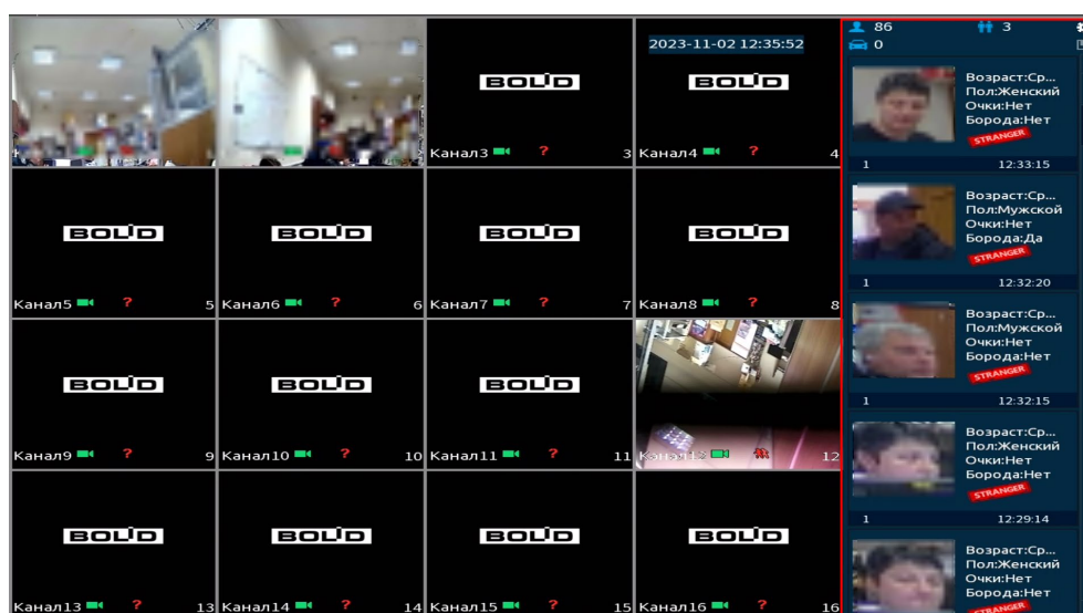
Рисунок 20.19 – Просмотр
