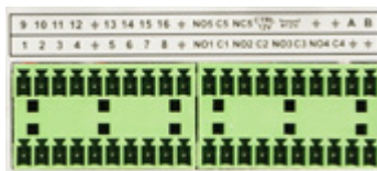
Рисунок 3.3 – Тревожный вход/выход, RS-485
