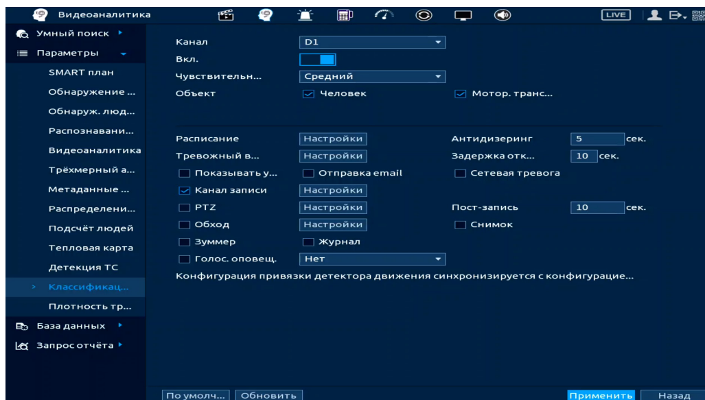
Рисунок 19.110 – Классификация объектов
