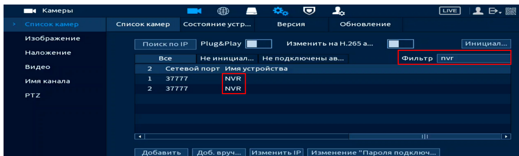
Рисунок 11.8 – Фильтр
