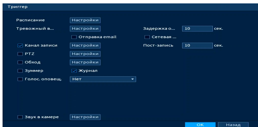
Рисунок 19.86 – Настройка
