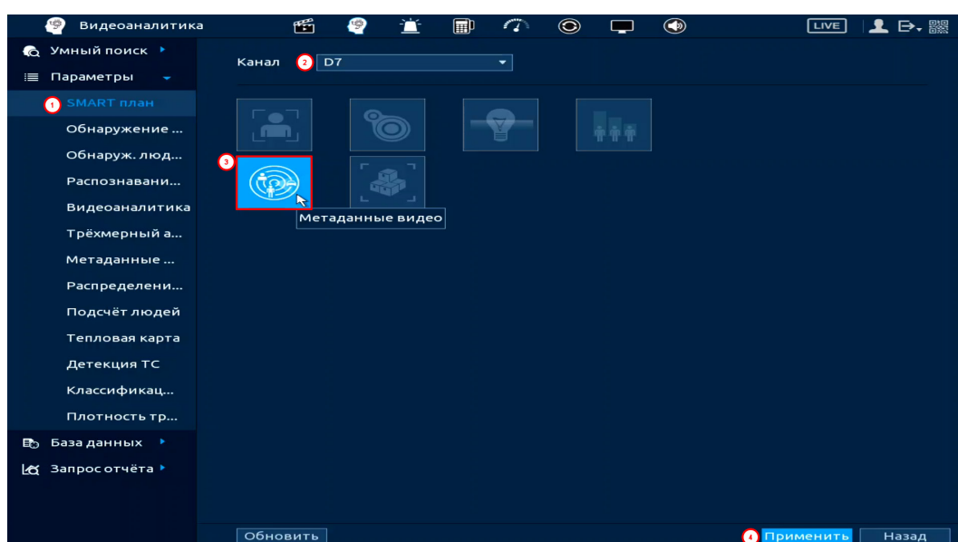
Рисунок 19.71 – Настройка
