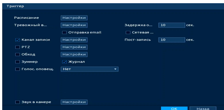
Рисунок 19.62 – Настройка
