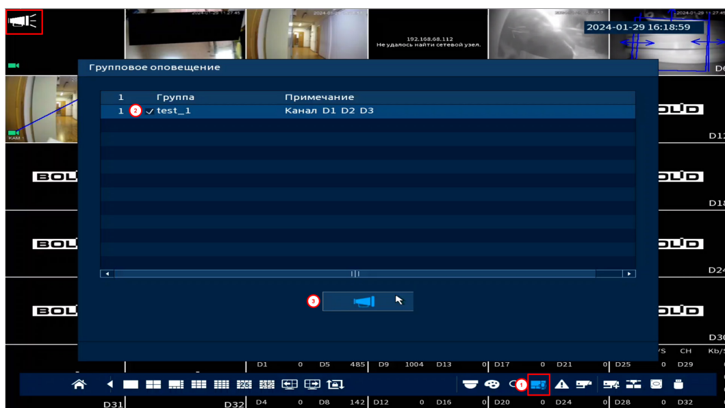
Рисунок 24.7 – Воспроизведение
