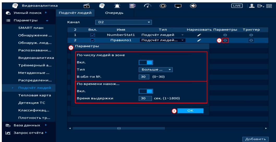
Рисунок 19.93 – Настройка параметров
