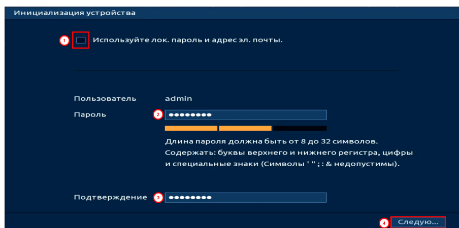
Рисунок 11.12 – Инициализация
