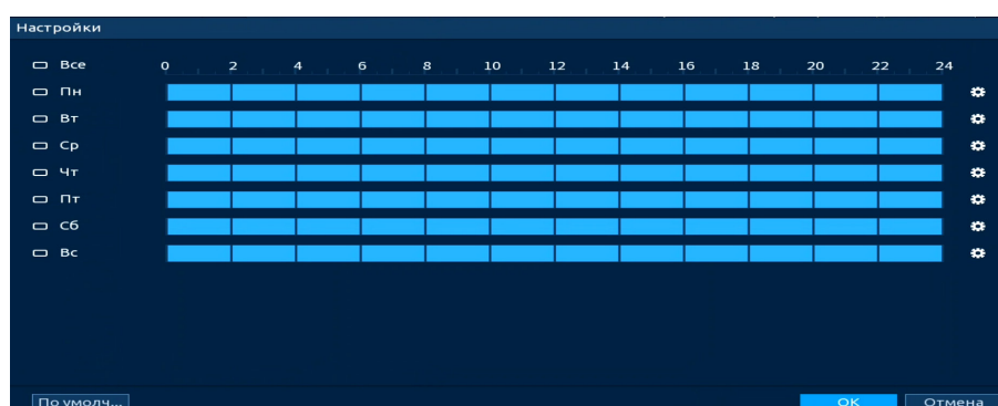
Рисунок 19.111 – Расписание
