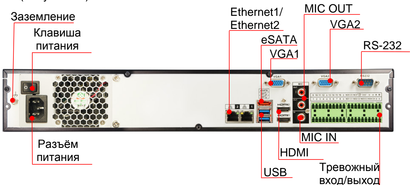
Рисунок 3.2 – Внешний вид задней панели
