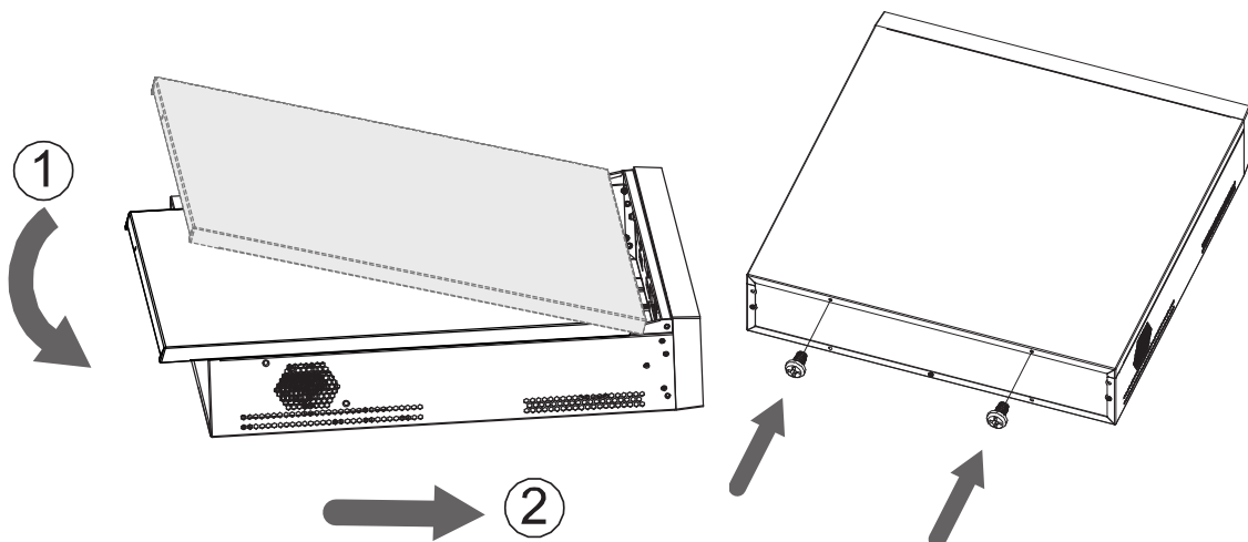
Рисунок 4.8 – Установка жёсткого диска
