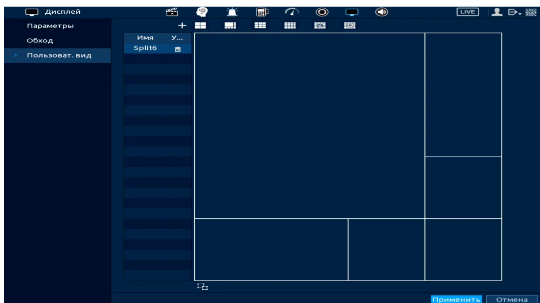
Рисунок 23.22 – Создание раскладки
