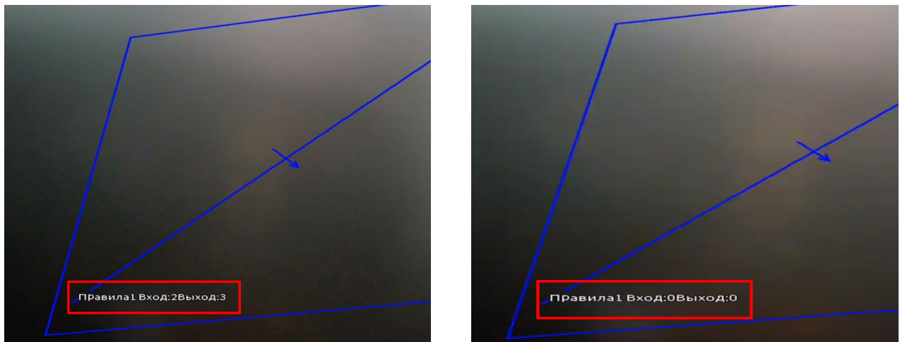
Рисунок 19.85 – Сброс
