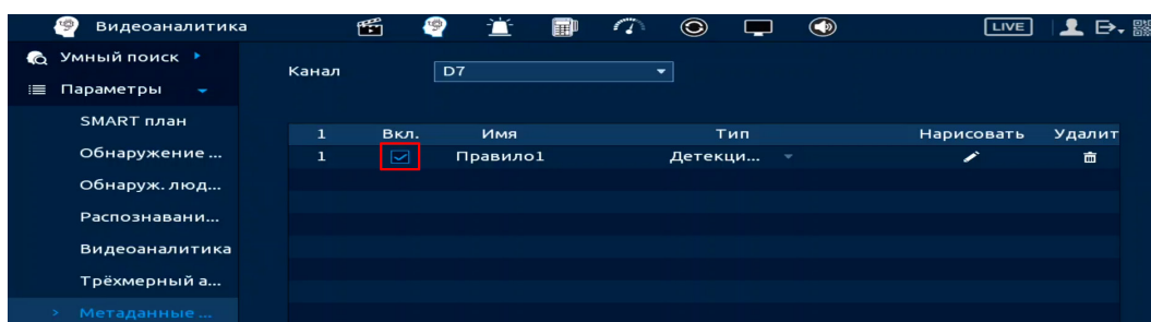
Рисунок 19.75 – Настройка
