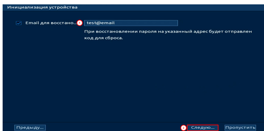
Рисунок 11.13 – Инициализация
