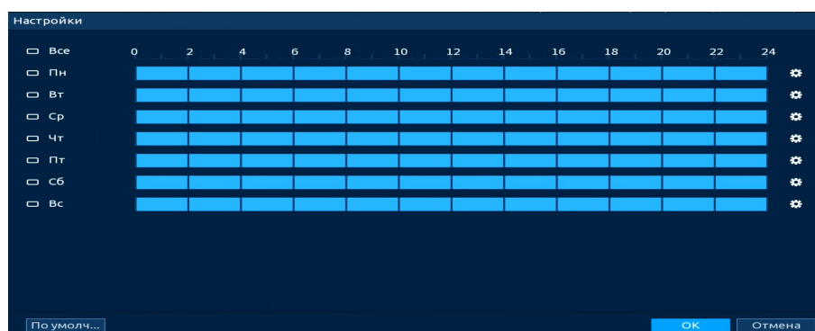
Рисунок 19.25 – Расписание
