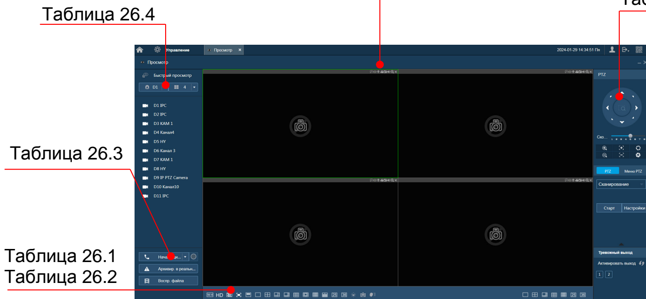
Рисунок 26.1 – Режим просмотра
