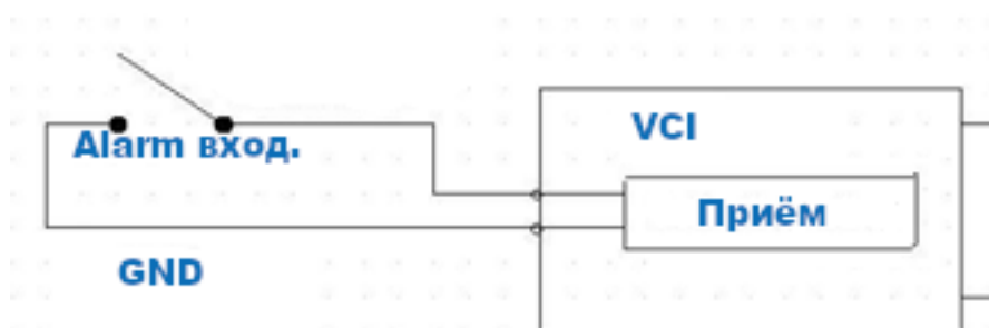
Рисунок 6.13 – Схема подключения тревожного входа
