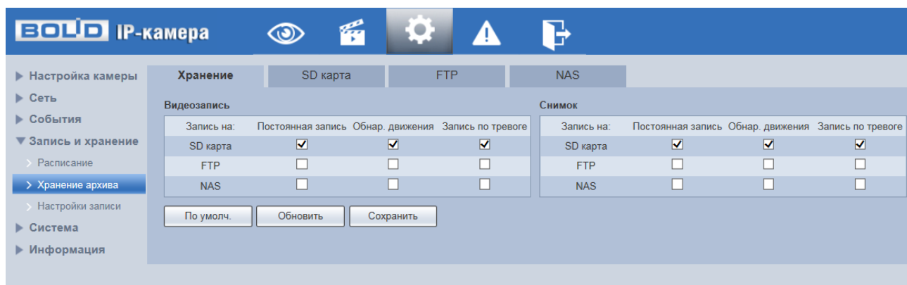
Рисунок 7.92 – Вкладка «Хранение»
