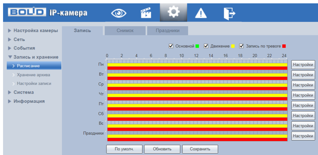
Рисунок 7.86 – Вкладка «Запись»
