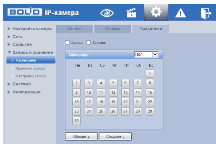
Рисунок 7.90 – Вкладка «Праздники»
