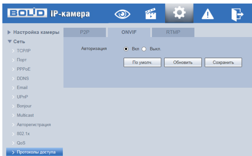
Рисунок 7.64 – Вкладка «ONVIF»
