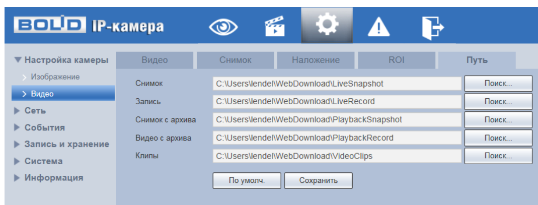
Рисунок 7.46 – Вкладка «Путь»
