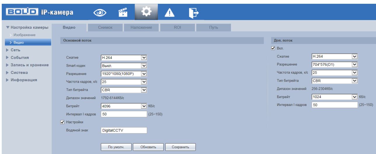
Рисунок 7.38 – Вкладка «Видео»
