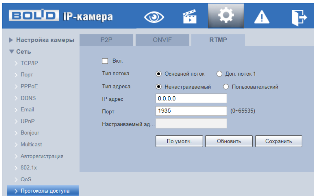
Рисунок 7.65 – Вкладка «RTMP»
