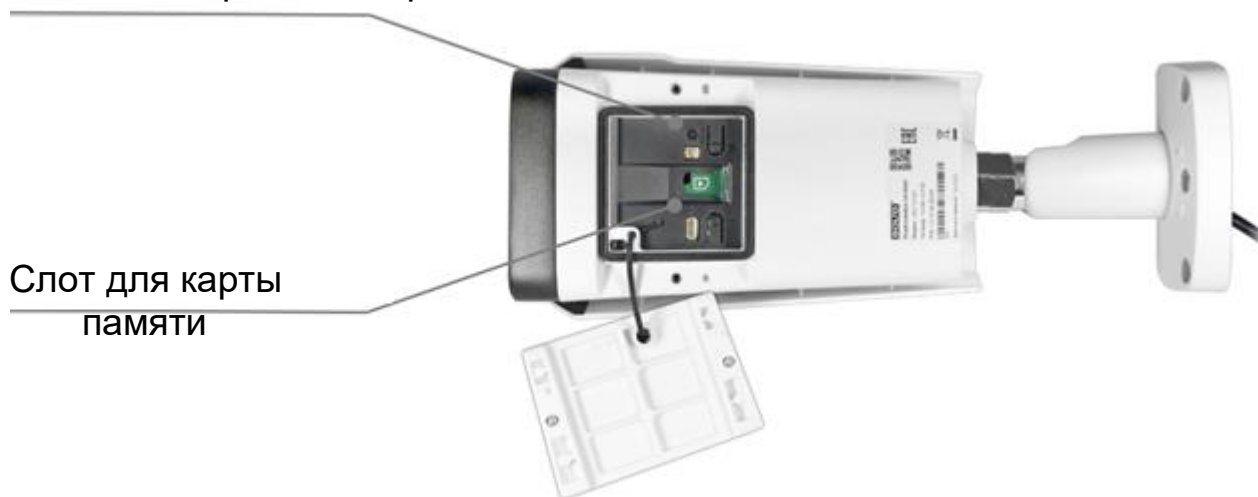
Рисунок 4.2 – Расположение кнопки аппаратного сброса и слота для карты памяти
