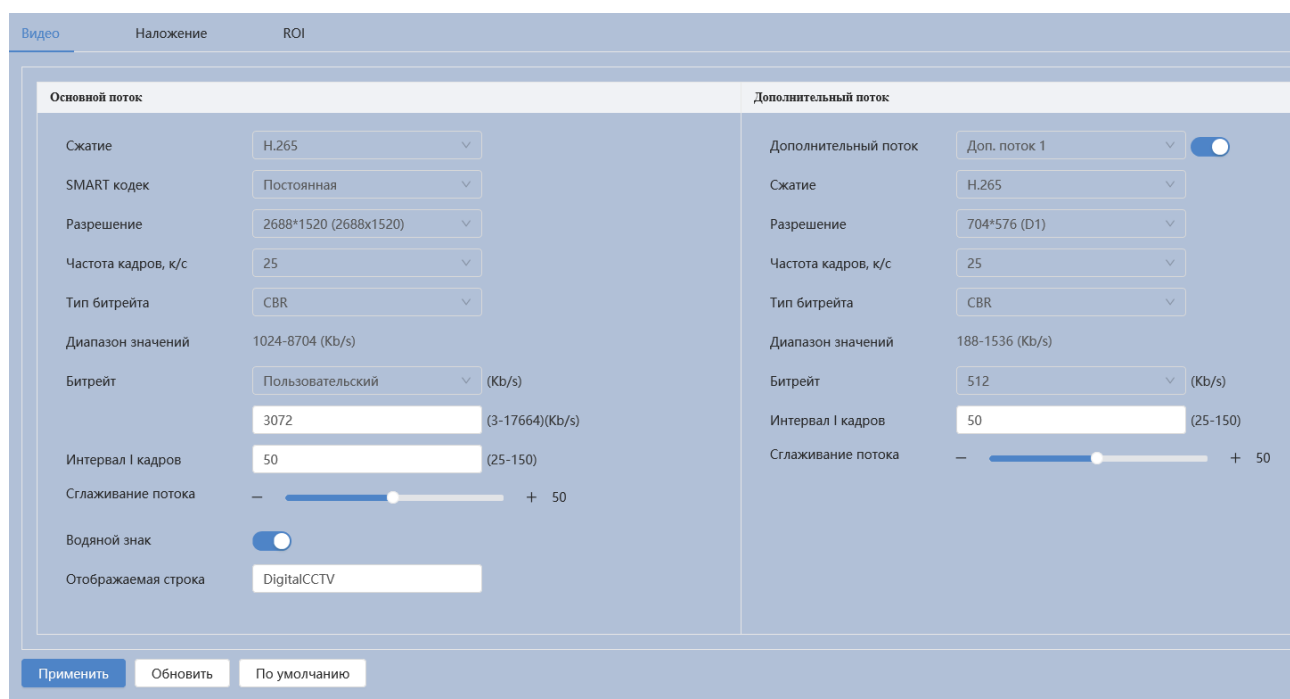
Рисунок 7.70 – Вкладка «Видео»
