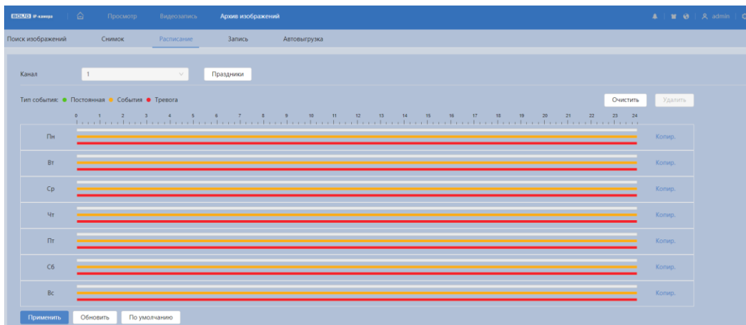
Рисунок 7.130 – Вкладка «Расписание»
