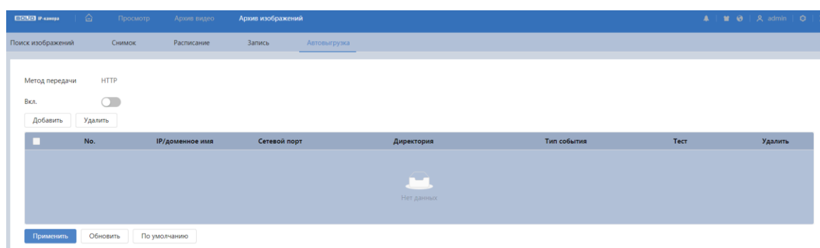
Рисунок 7.134 – Вкладка «Автовыгрузка»
