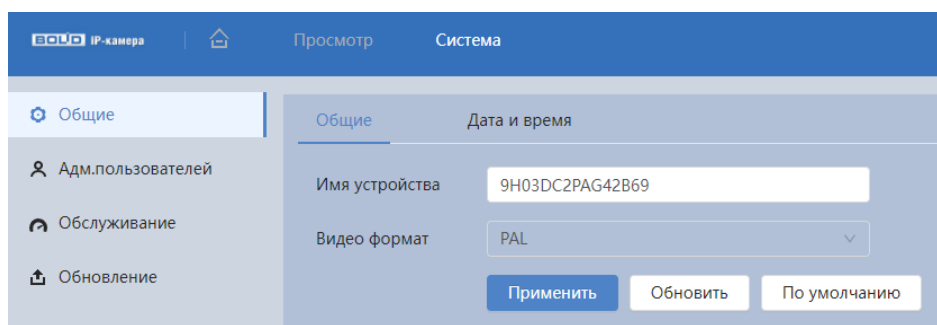
Рисунок 7.102 – Вкладка «Общие»
