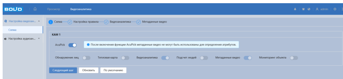
Рисунок 7.23 – Функция «АсуРiск»
