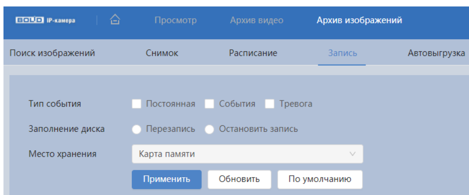
Рисунок 7.132 – Вкладка «Запись»
