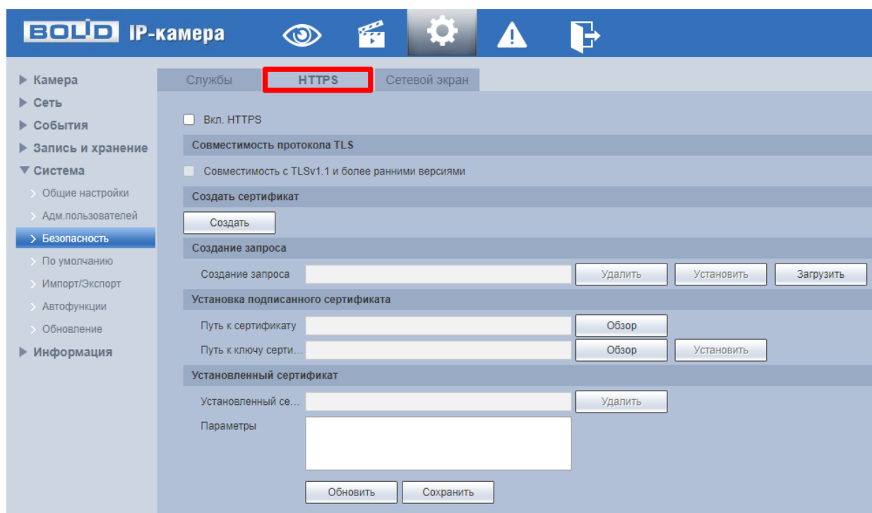
Рисунок 7.121 – Вкладка «HTTPS»
