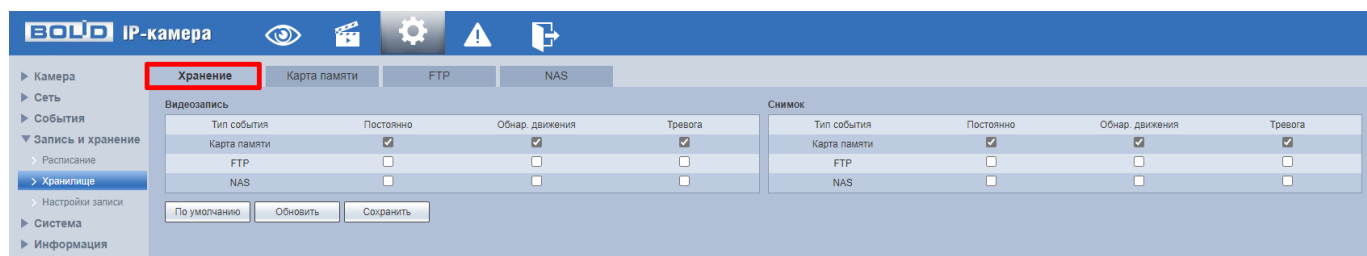
Рисунок 7.106 – Вкладка «Хранение»
