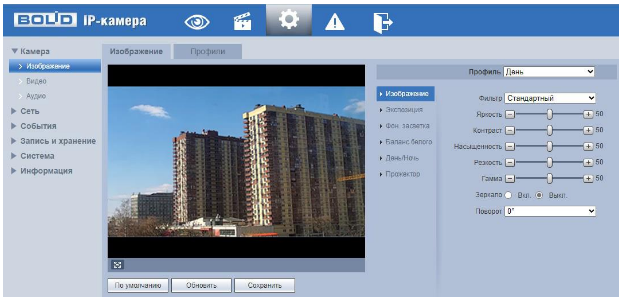
Рисунок 7.27 – Вкладка «Изображение»
