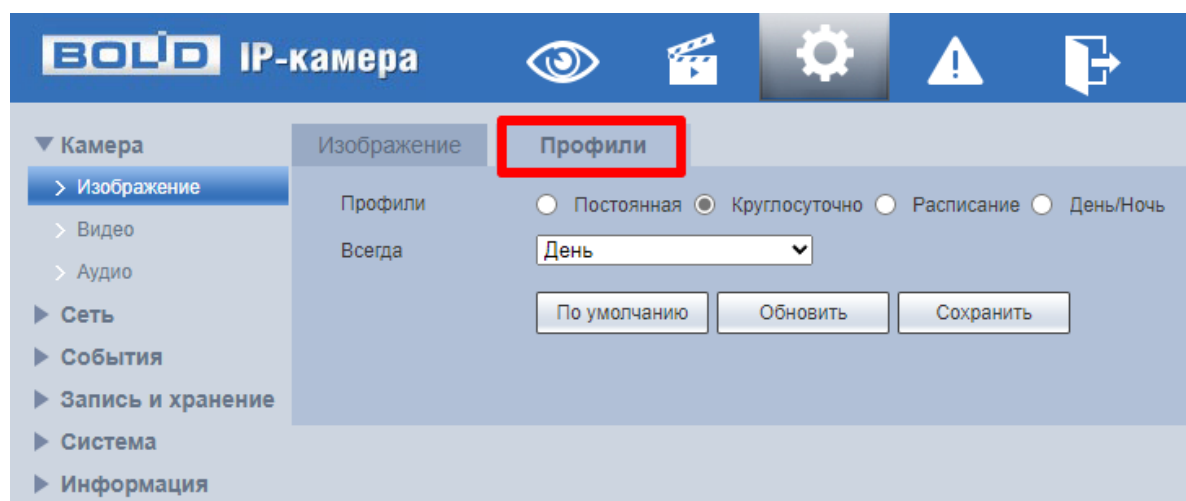
Рисунок 7.36 – Вкладка «Профили»
