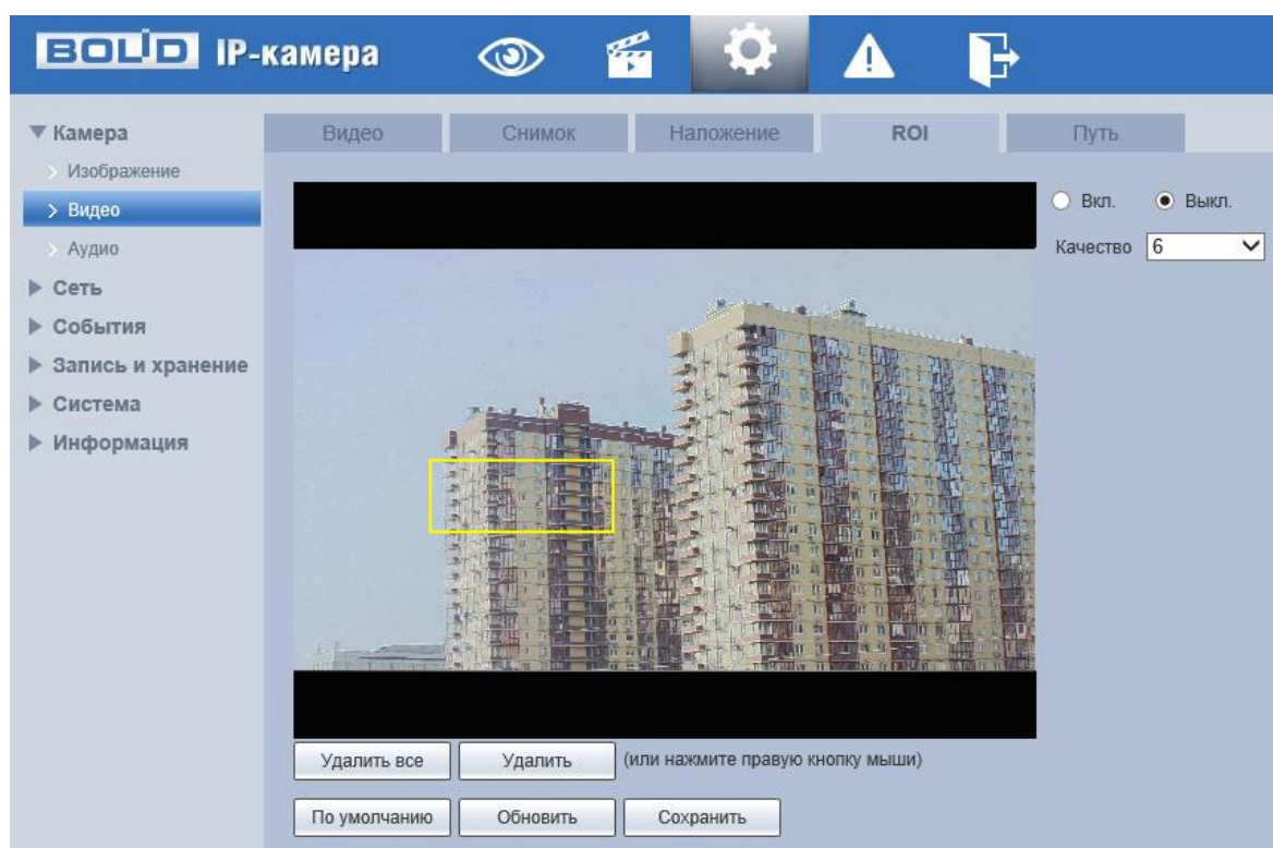
Рисунок 7.47 – Вкладка «ROI»
