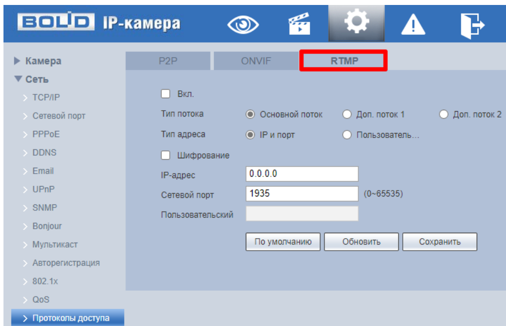
Рисунок 7.70 – Вкладка «RTMP»
