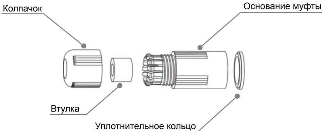
Рисунок 6.5 – Элементы герметичной кабельной муфты
