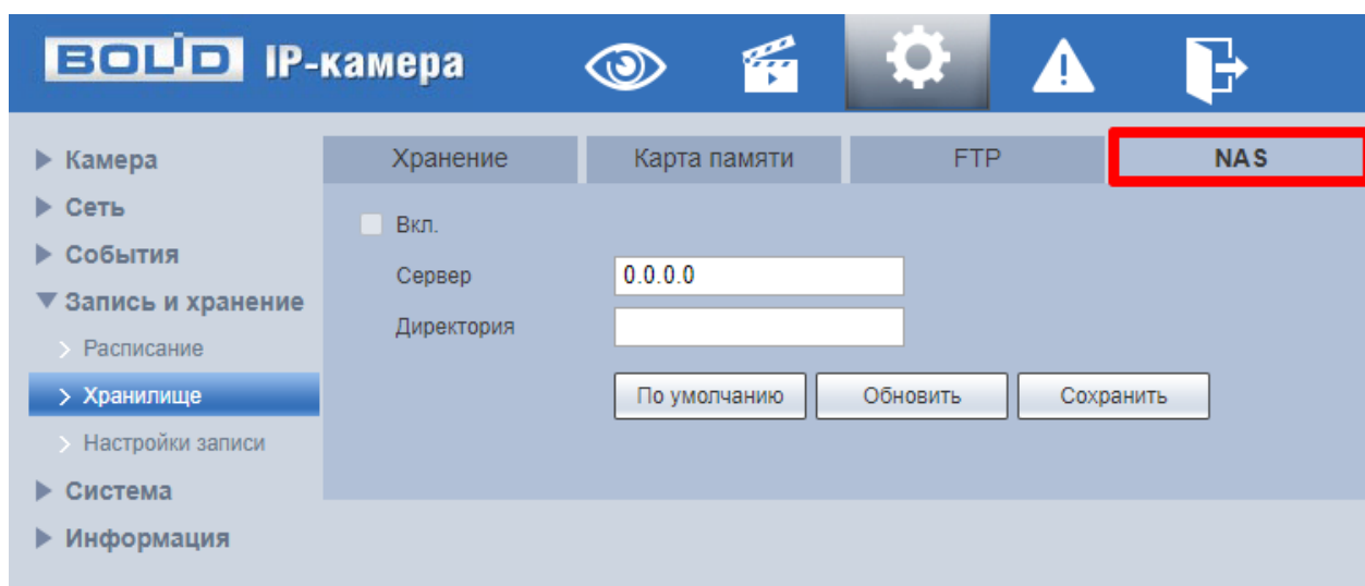
Рисунок 7.109 – Вкладка «NAS»
