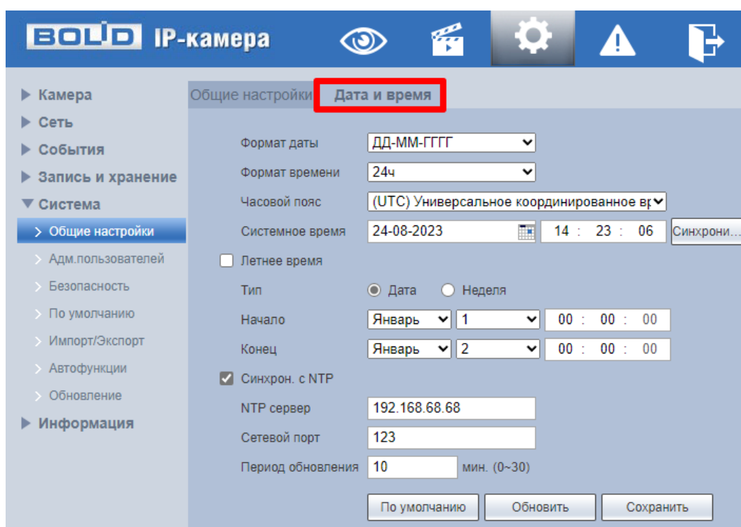
Рисунок 7.115 – Вкладка «Дата/Время»
