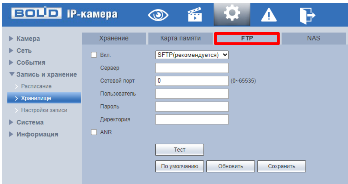
Рисунок 7.108 – Вкладка «FTP»
