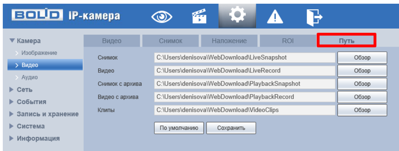
Рисунок 7.48 – Вкладка «Путь»
