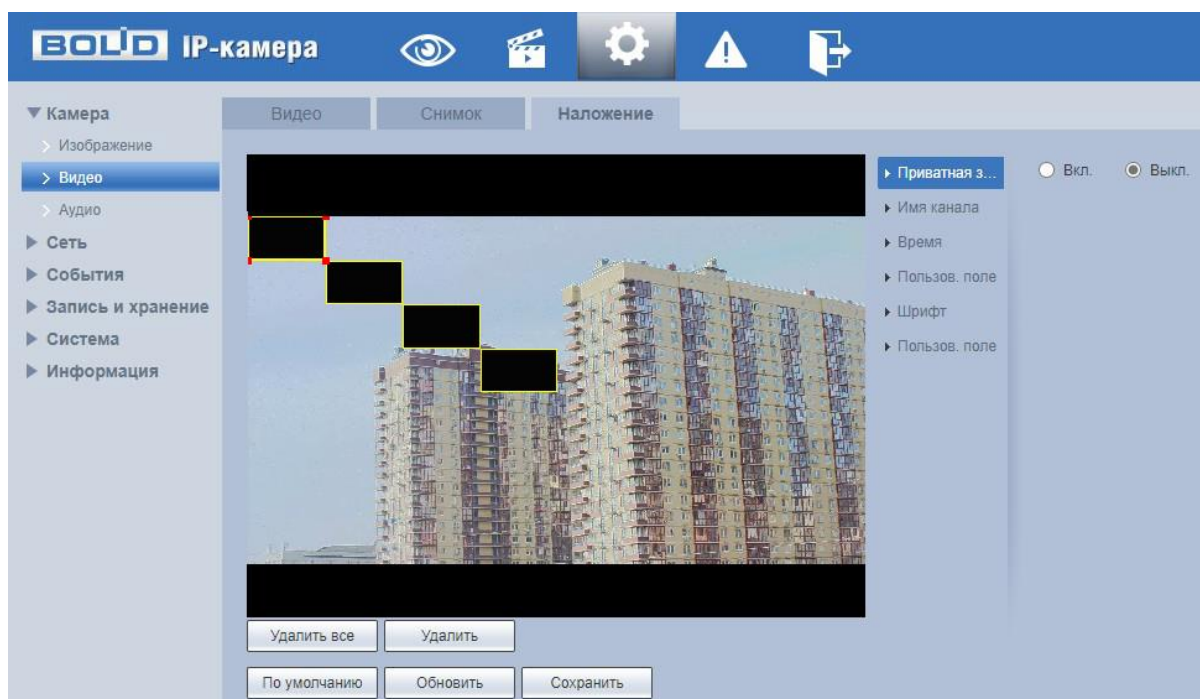
Рисунок 7.40 – Вкладка «Наложение»
