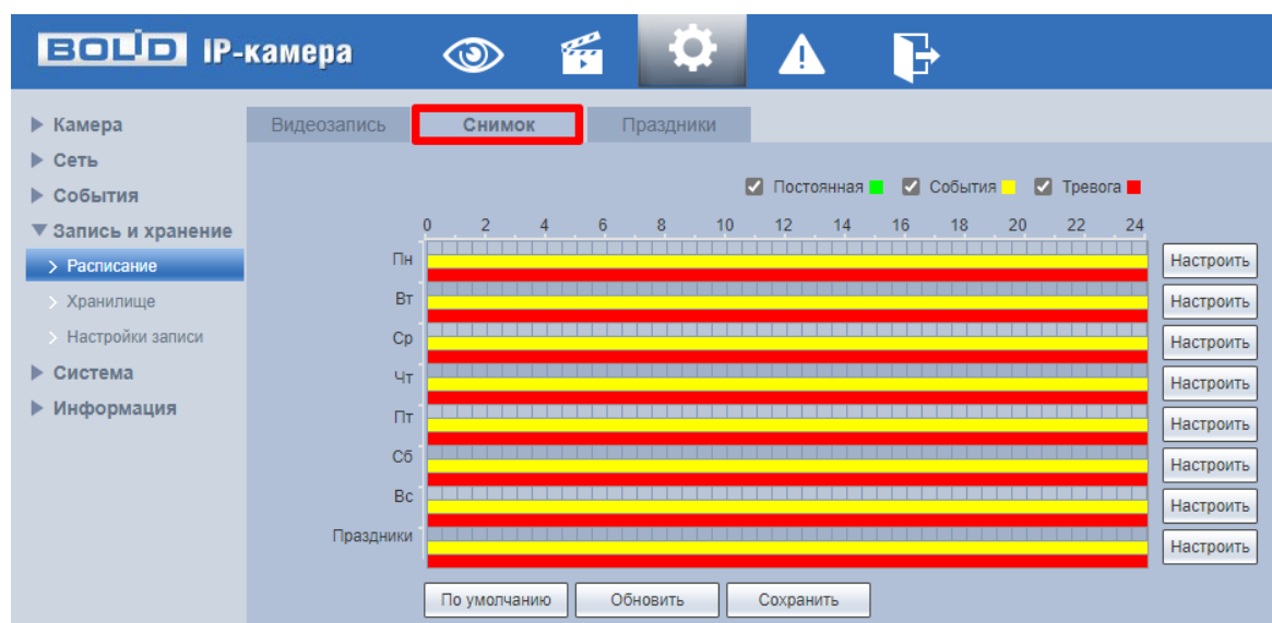
Рисунок 7.102 – Вкладка «Снимок»
