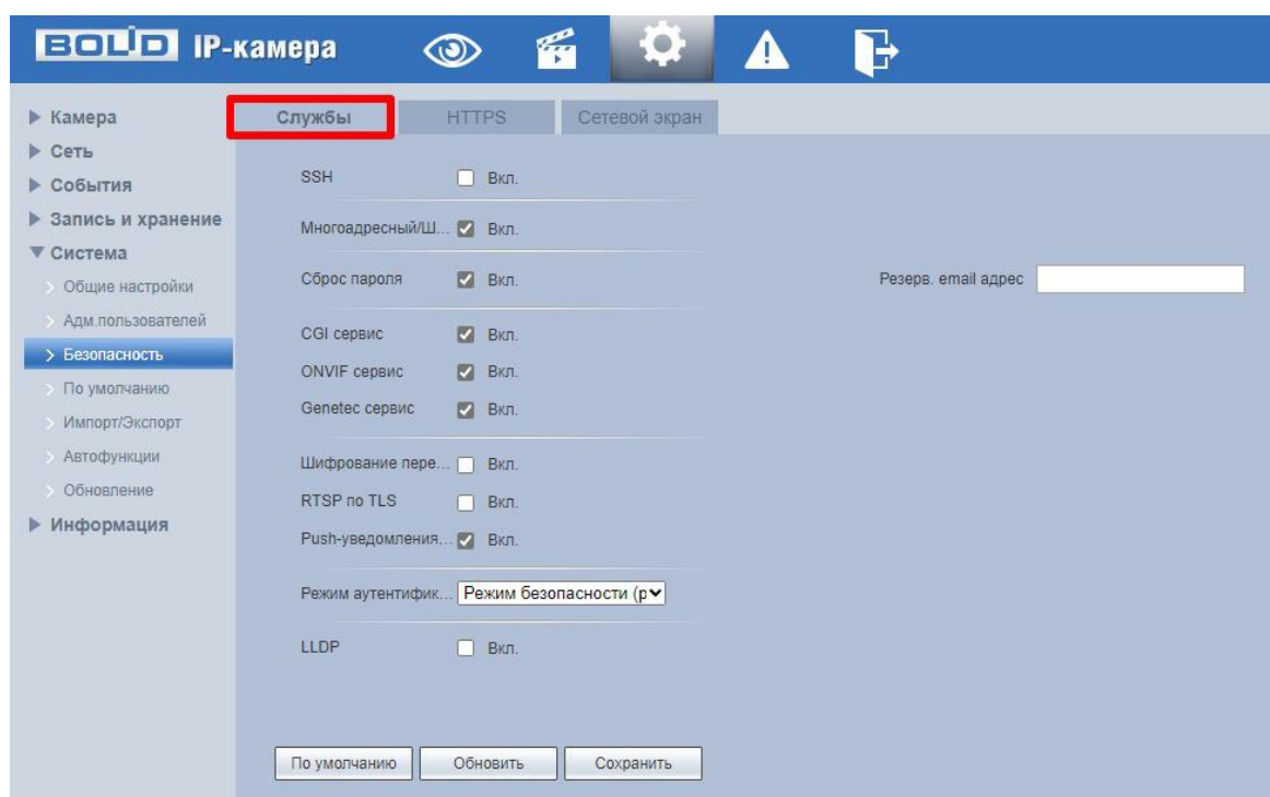
Рисунок 7.120 – Вкладка «Службы»
