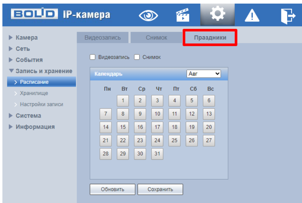
Рисунок 7.104 – Вкладка «Праздники»
