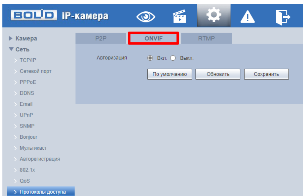
Рисунок 7.69 – Вкладка «ONVIF»
