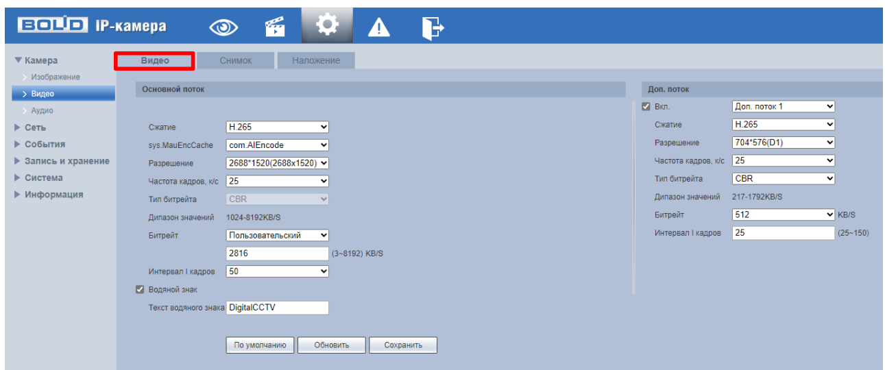
Рисунок 7.38 – Вкладка «Видео»
