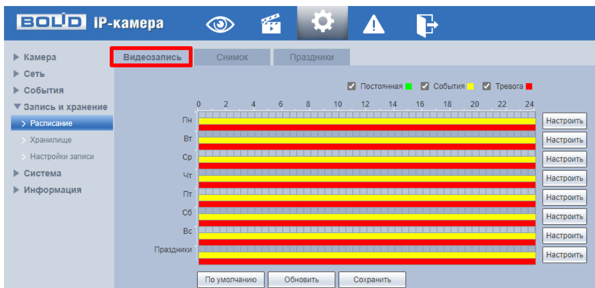
Рисунок 7.100 – Вкладка «Видеозапись»
