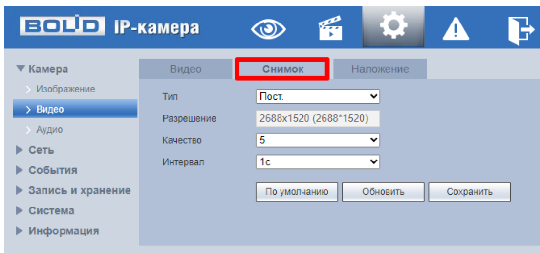
Рисунок 7.39 – Вкладка «Снимок»
