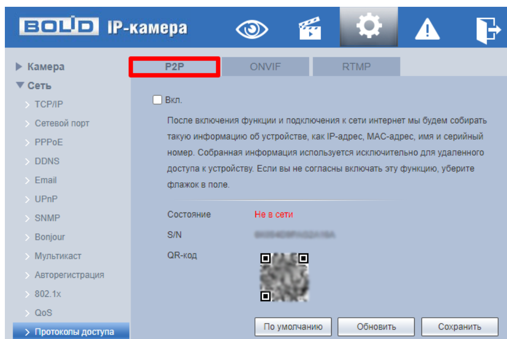
Рисунок 7.68 – Вкладка «P2P»
