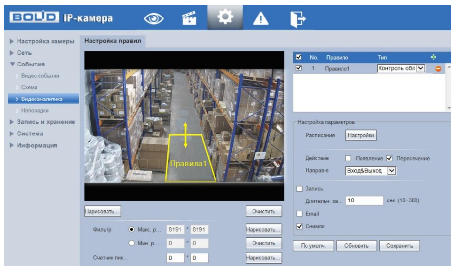
Рисунок 7.85 – Создание правила видеоаналитики «Контроль области»
