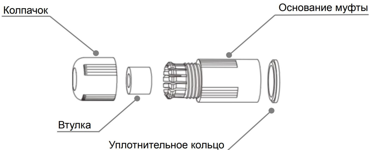
Рисунок 6.5 – Элементы герметичной кабельной муфты
