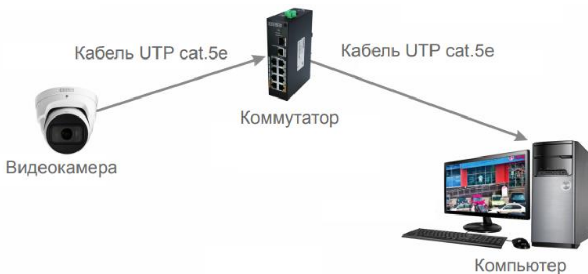
Рисунок 6.3 – Схема подключения видеокамеры к компьютеру через коммутатор
