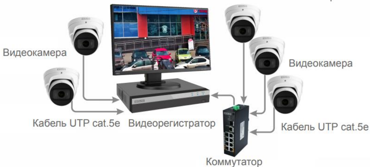
Рисунок 6.4 – Схема подключения видеокамеры к видеорегистратору
