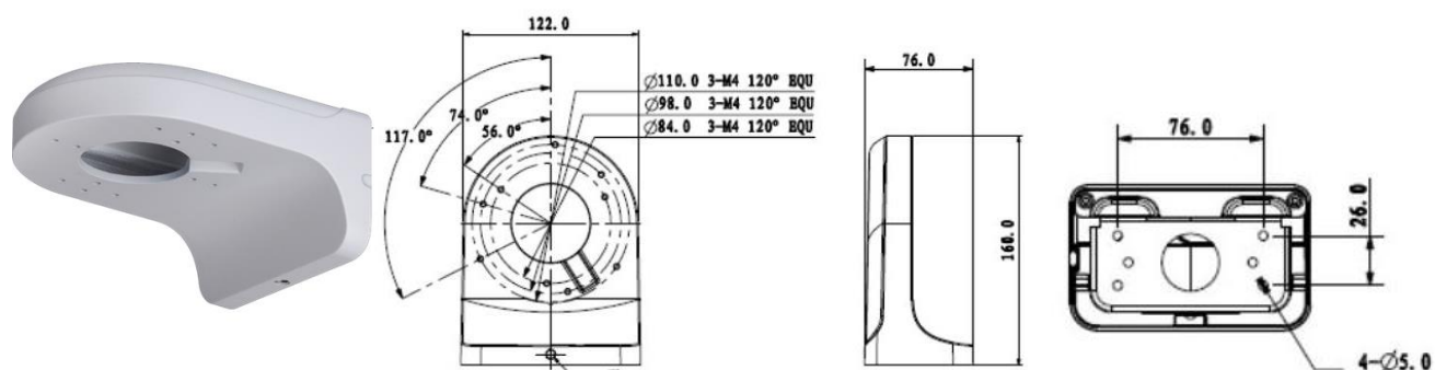
Рисунок 5.7 – Внешний вид и габаритные размеры кронштейна BR-106
