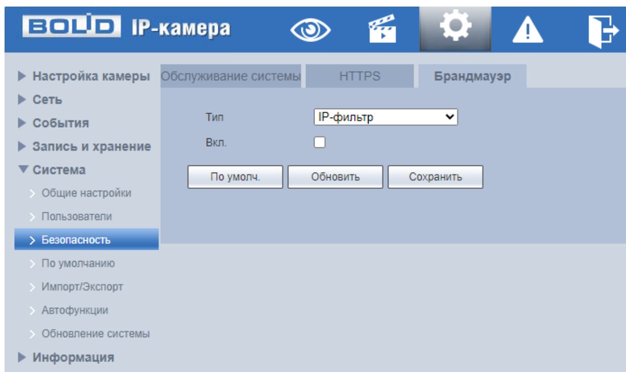
Рисунок 7.121 – Вкладка «Брандмауэр»
