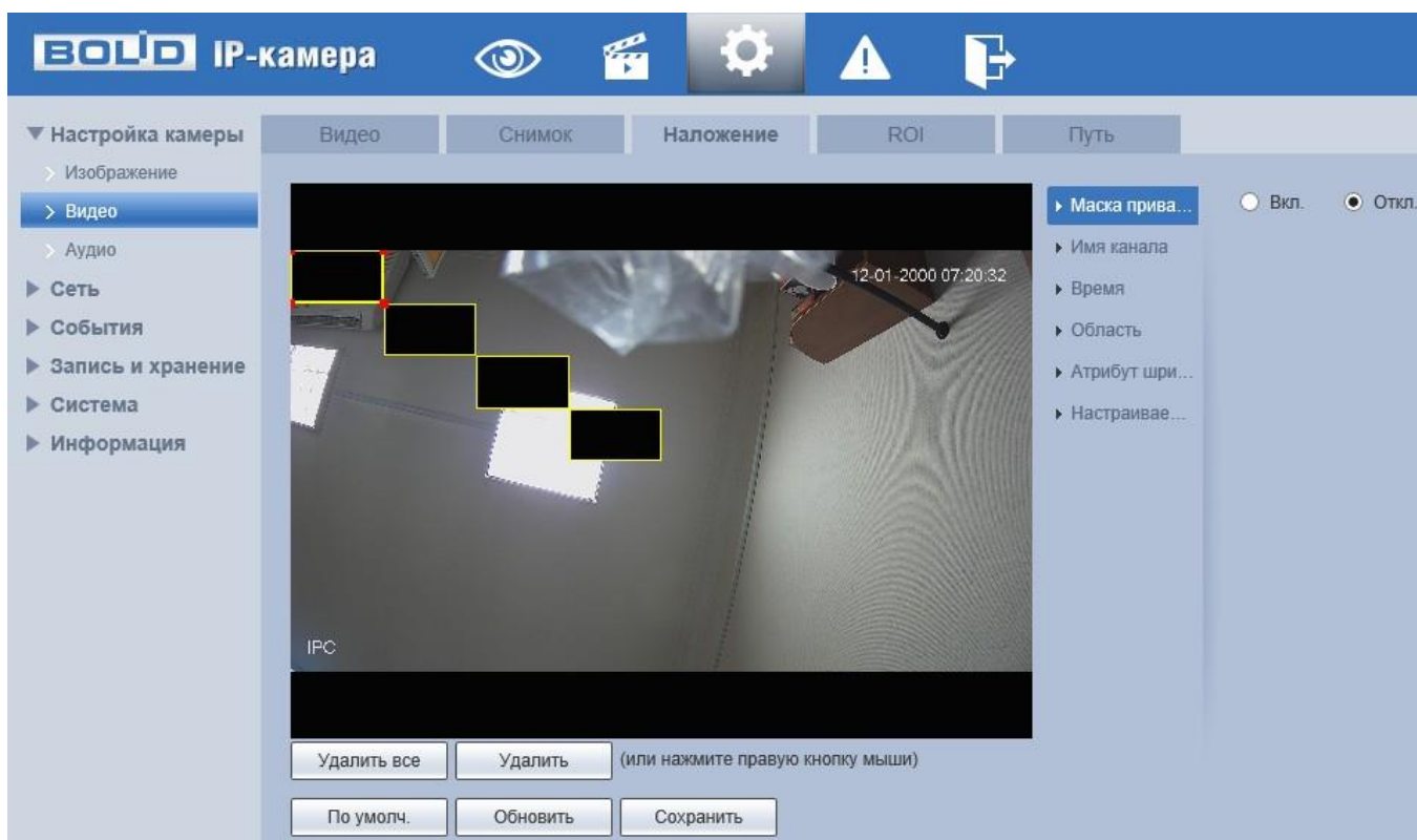
Рисунок 7.41 – Вкладка «Наложение»
