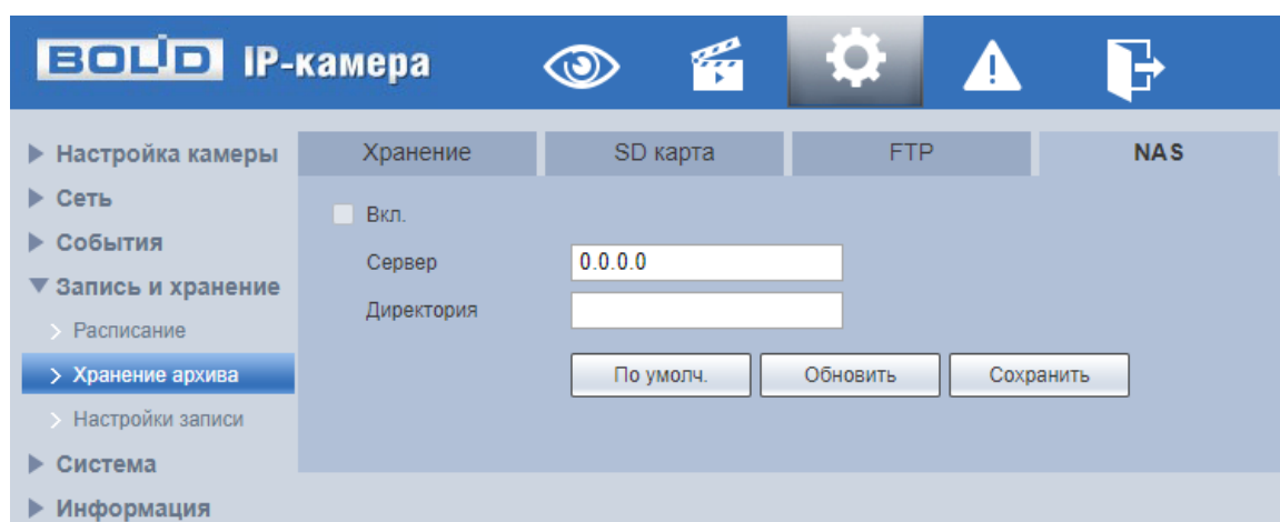
Рисунок 7.107 – Вкладка «NAS»
