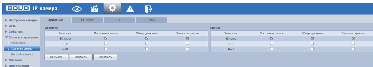
Рисунок 7.104 – Вкладка «Хранение»
