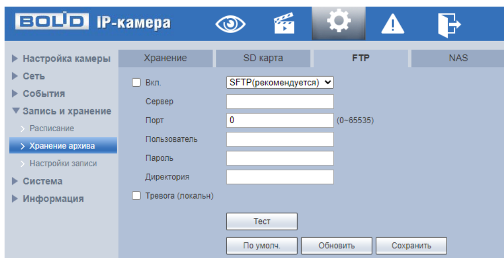
Рисунок 7.106 – Вкладка «FTP»
