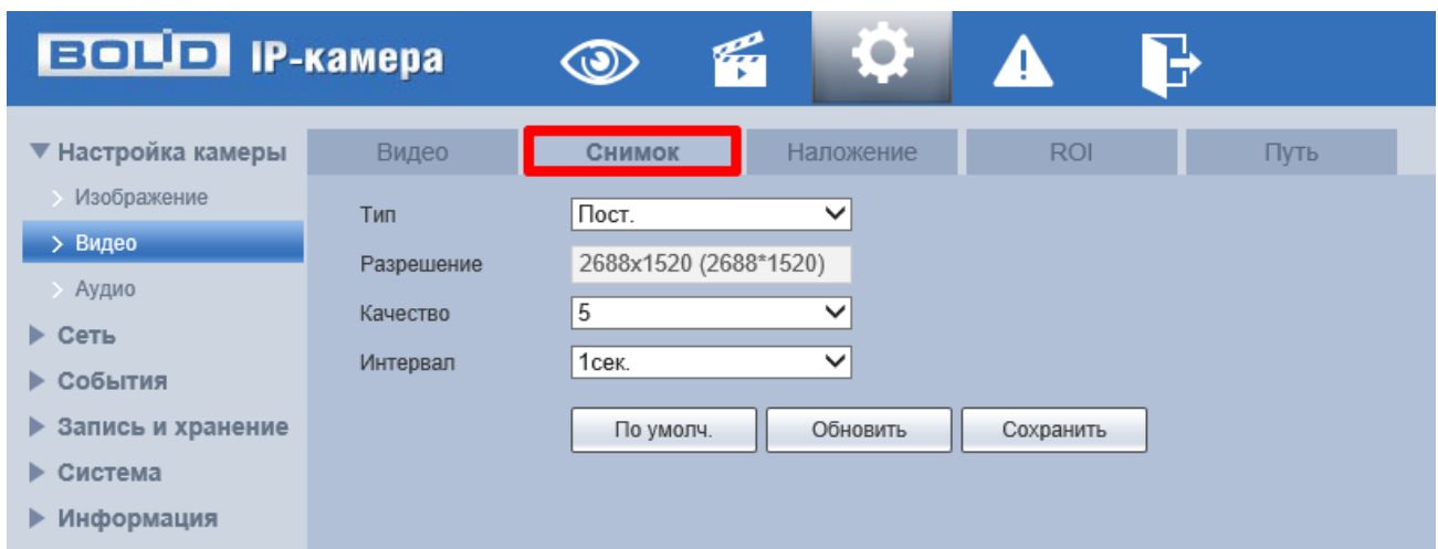
Рисунок 7.40 – Вкладка «Снимок»
