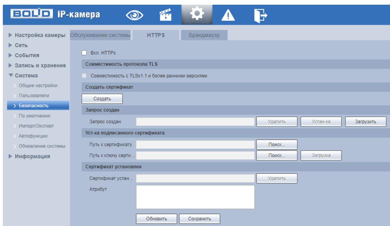
Рисунок 7.119 – Вкладка «HTTPS»
