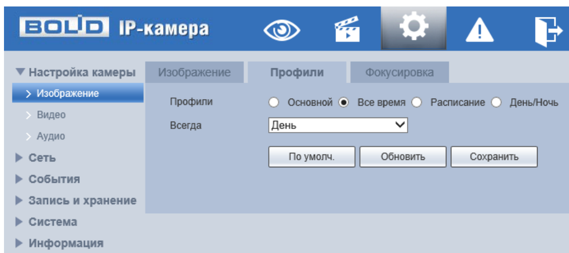
Рисунок 7.36 – Вкладка «Профили»
