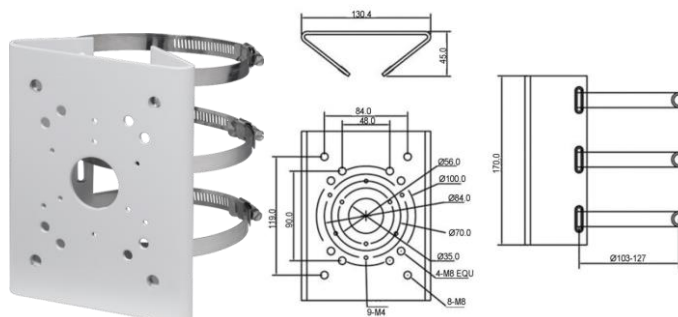
Рисунок 5.13 – Столбовой кронштейн BR-103
