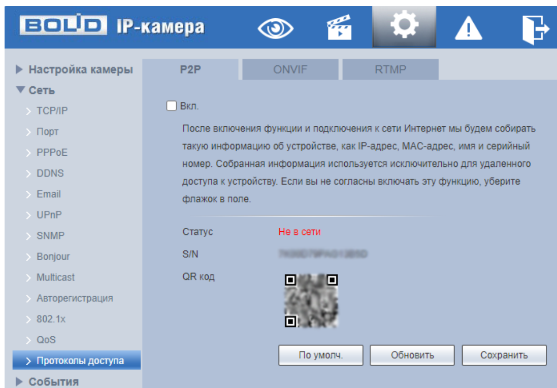
Рисунок 7.69 – Вкладка «P2P»
