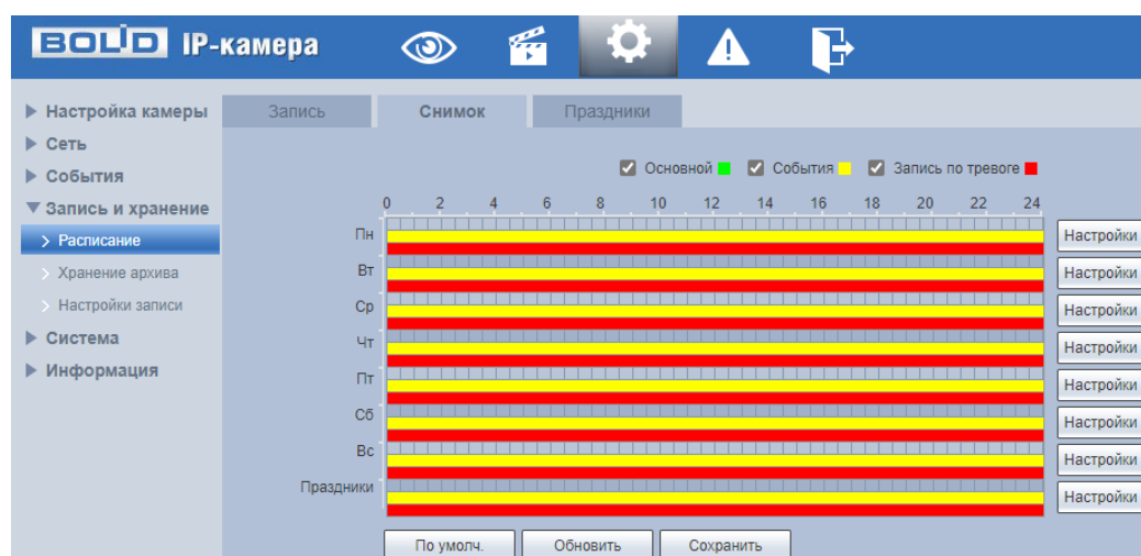
Рисунок 7.100 – Вкладка «Снимок»
