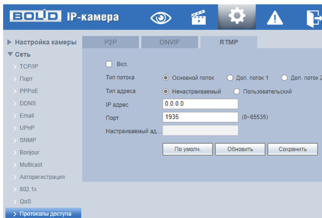
Рисунок 7.71 – Вкладка «RTMP»
