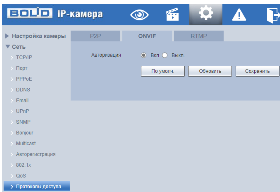
Рисунок 7.70 – Вкладка «ONVIF»
