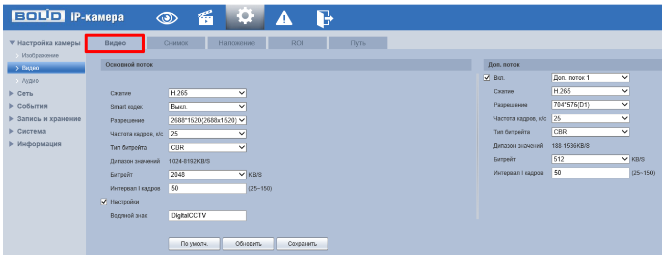
Рисунок 7.39 – Вкладка «Видео»
