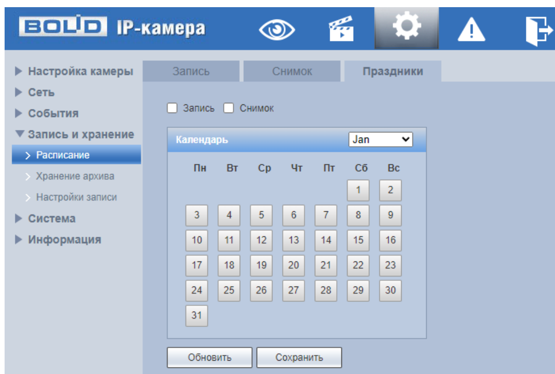
Рисунок 7.102 – Вкладка «Праздники»
