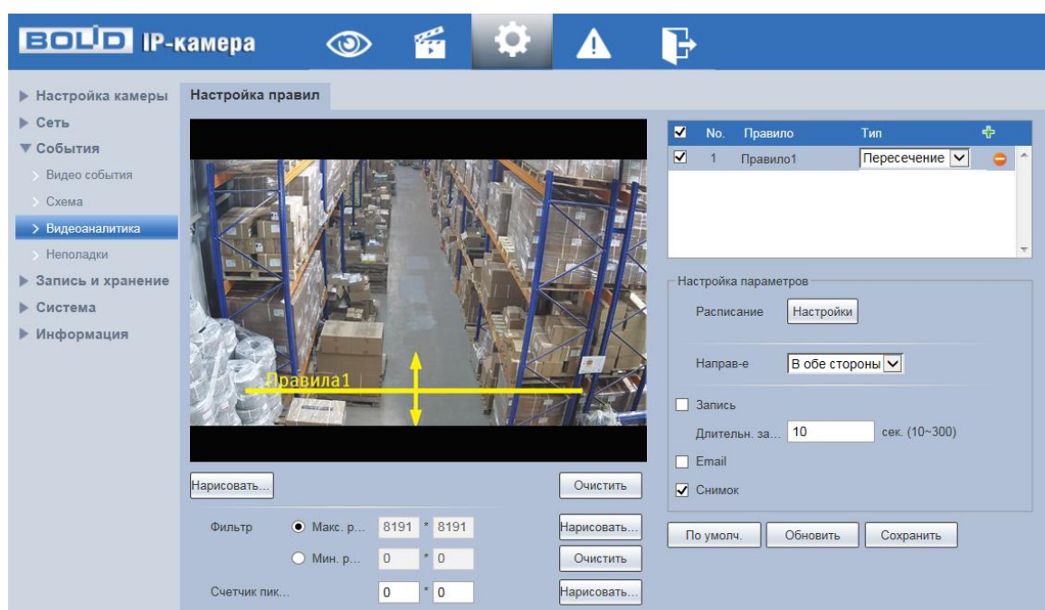
Рисунок 7.82 – Создание правила видеоаналитики «Пересечение линии»
