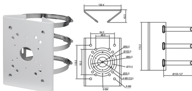
Рисунок 5.13 – Столбовой кронштейн BR-103
