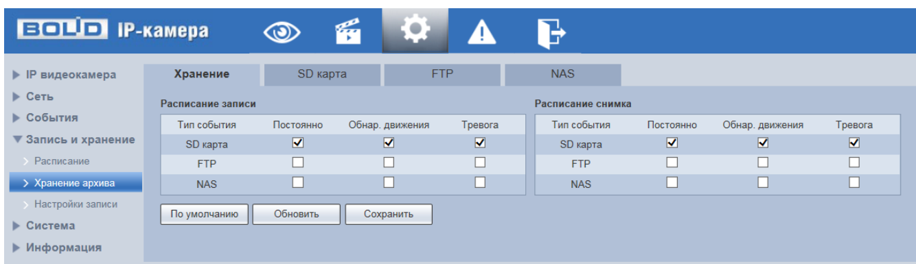
Рисунок 7.99 – Вкладка «Хранение»
