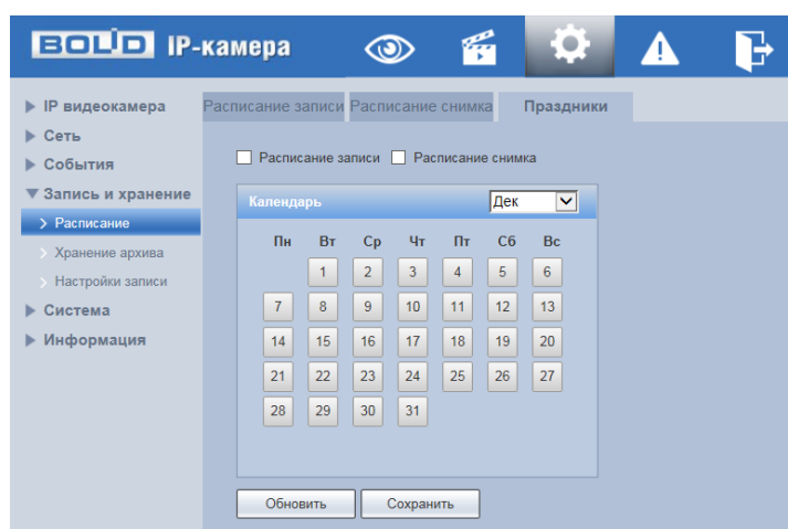
Рисунок 7.97 – Вкладка «Праздники»
