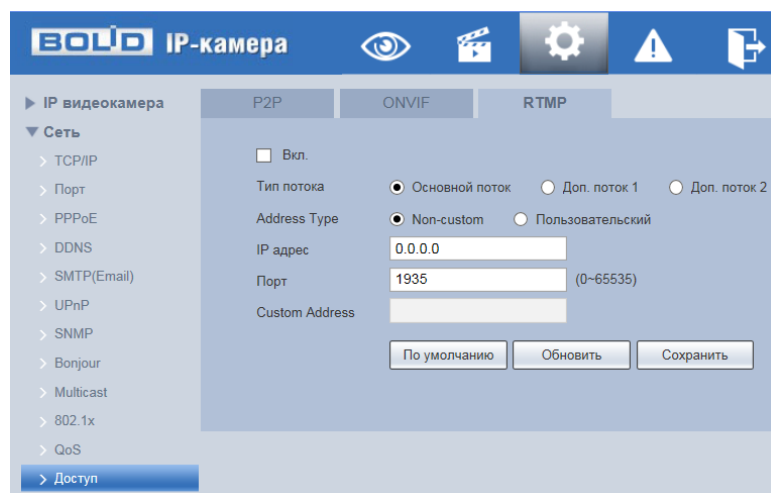
Рисунок 7.68 – Вкладка «RTMP»
