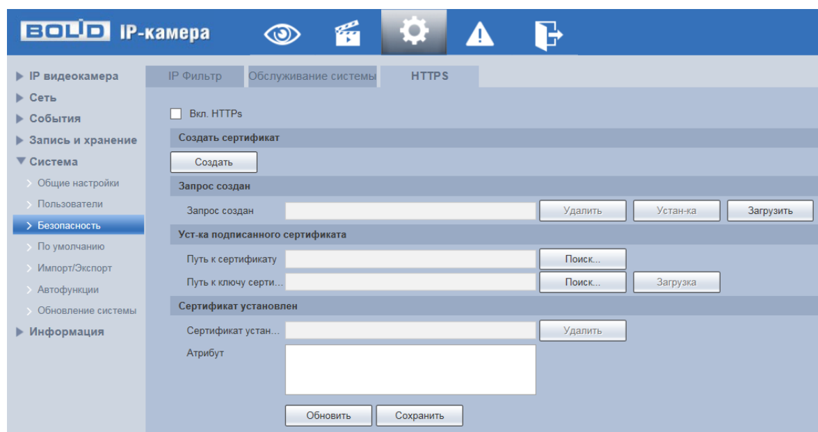
Рисунок 7.116 – Вкладка «HTTPS»
