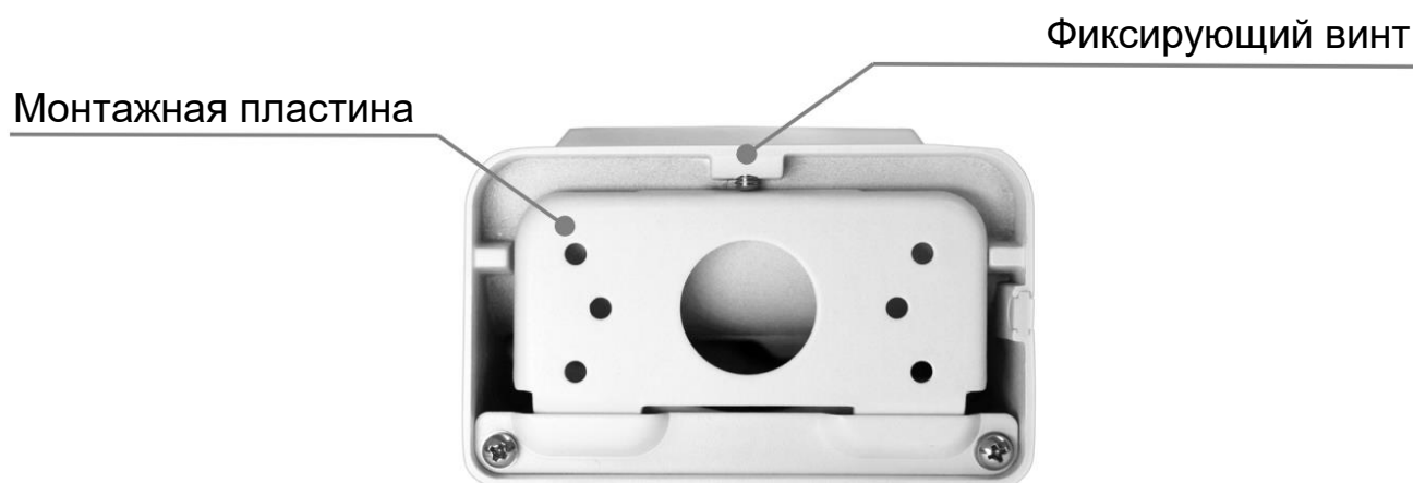
Рисунок 5.8 – Настенный кронштейн
