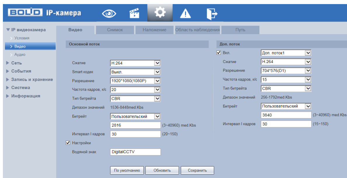
Рисунок 7.38 – Вкладка «Видео»
