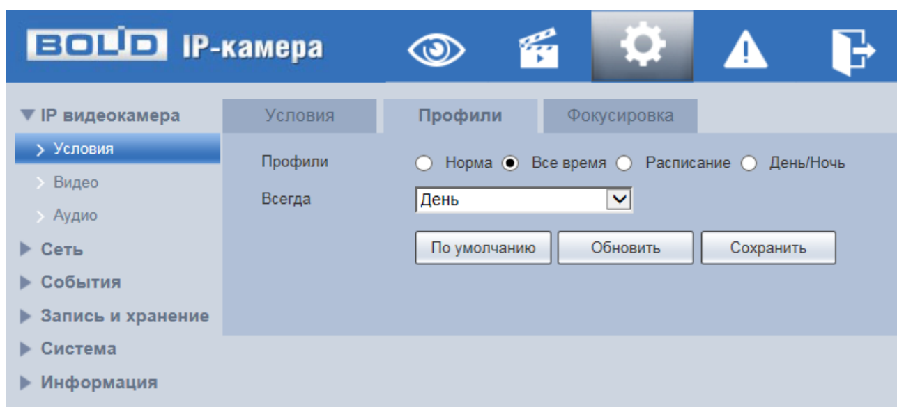
Рисунок 7.36 – Вкладка «Профили»
