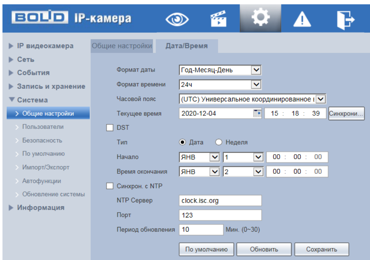
Рисунок 7.108 – Вкладка «Дата/Время»
