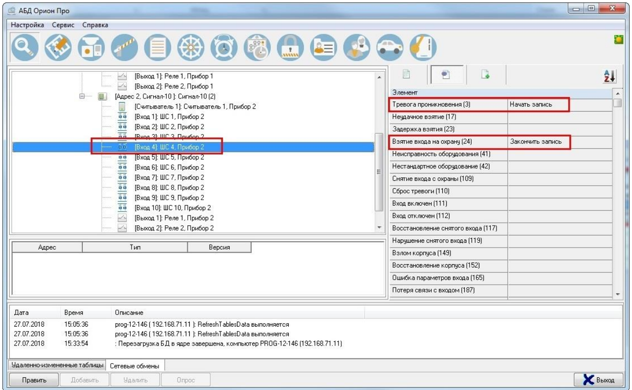
Рисунок 3-106 Реализация запуска и завершения записи по событиям объекта "Вход"
